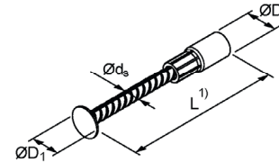
Bild 4: Kompaktanker
