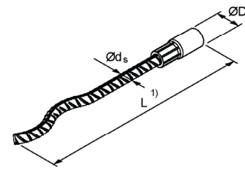
Bild 5: Gewindeanker gewellt
